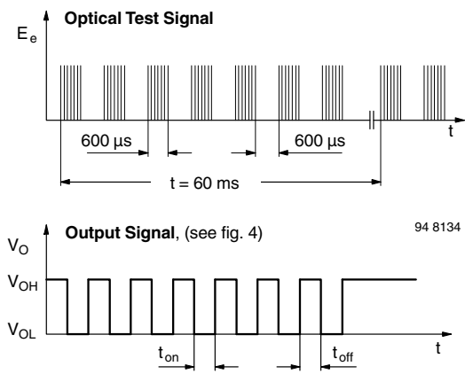
Fig. 3 - Output Function
