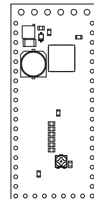
5 Actual size Scale 1:1
