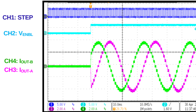
Output Enabled
