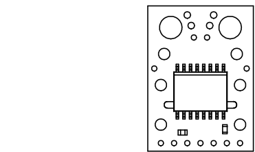
5 Actual size Scale 1:1
