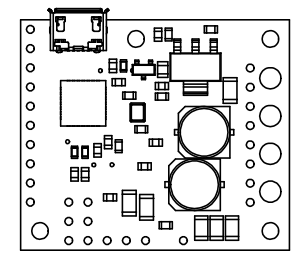
⑤ Actual size Scale 1:1
