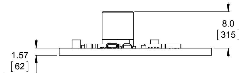
4 Profile Scale 2:1
